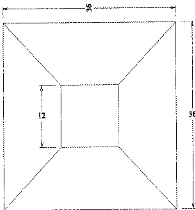
CLCC36 COLUMN CAP
